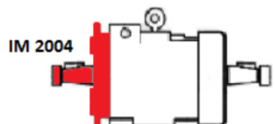
Лапы / Фланец. Два конических вала
