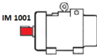
Лапы. Цилиндрический вал
